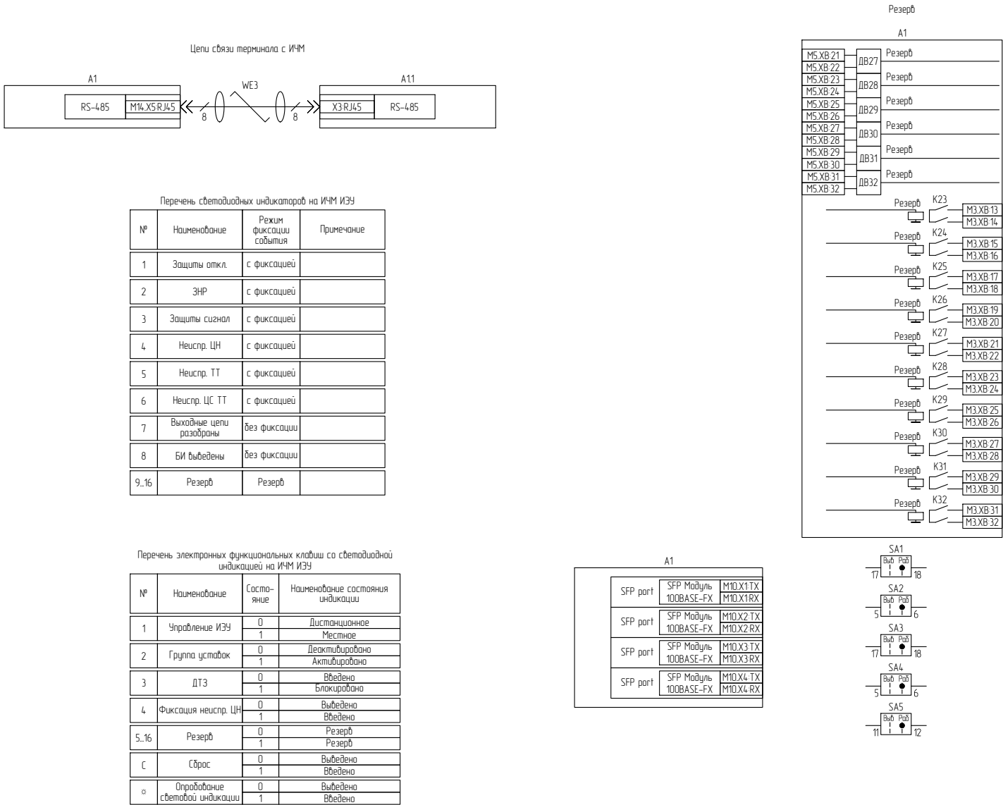
Рисунок Г.4 – Схема электрическая принципиальная (часть 4)
